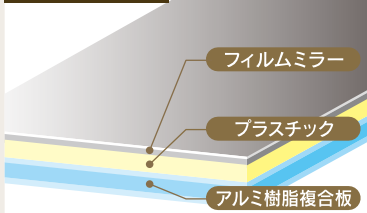
ミラー断面図
