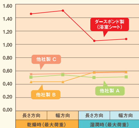
■摩擦比較測定データグラフ(単位:kg)
